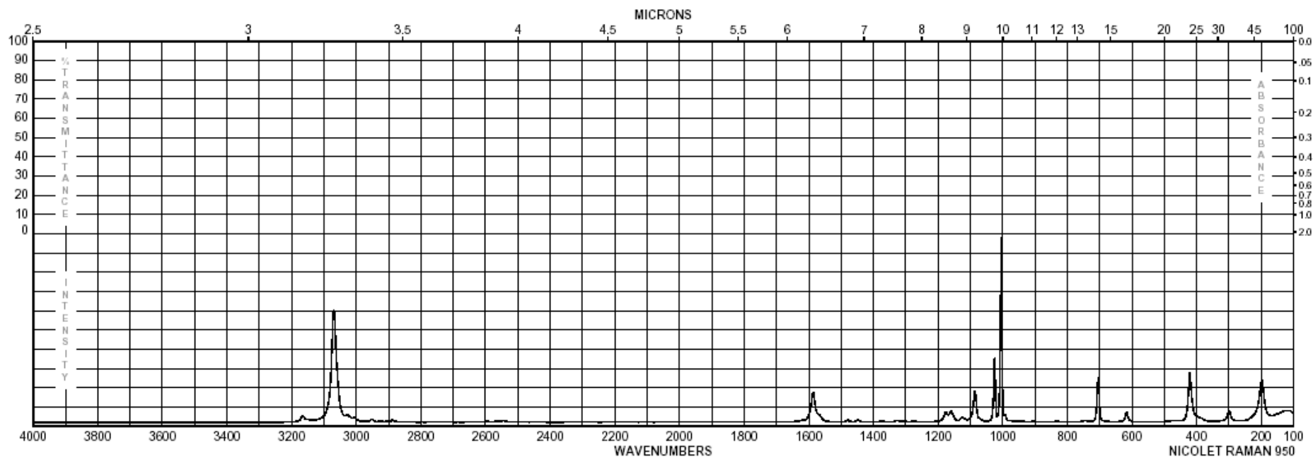
氯苯
