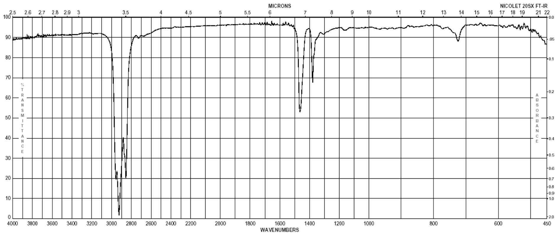
石蜡油
