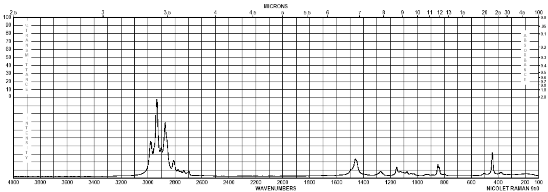
乙醚
