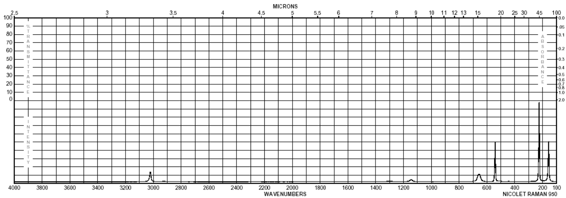
三溴甲烷
