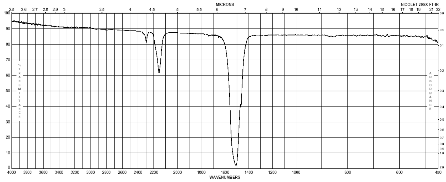
二硫化碳
