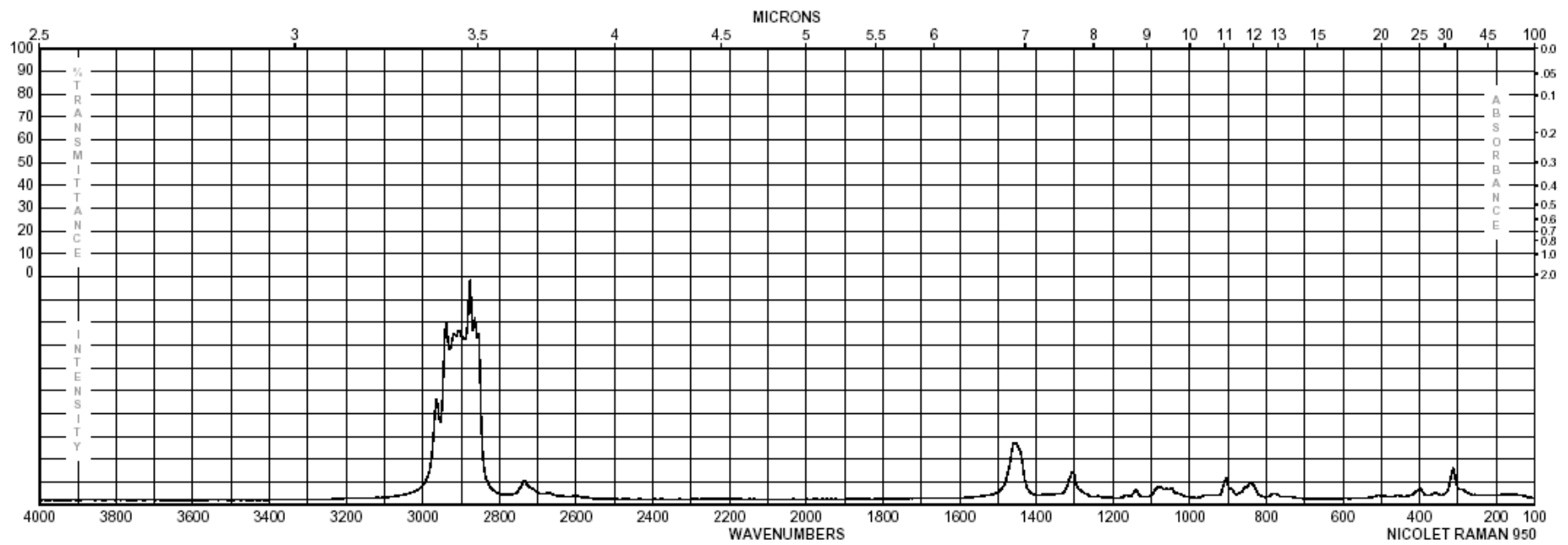
正庚烷
