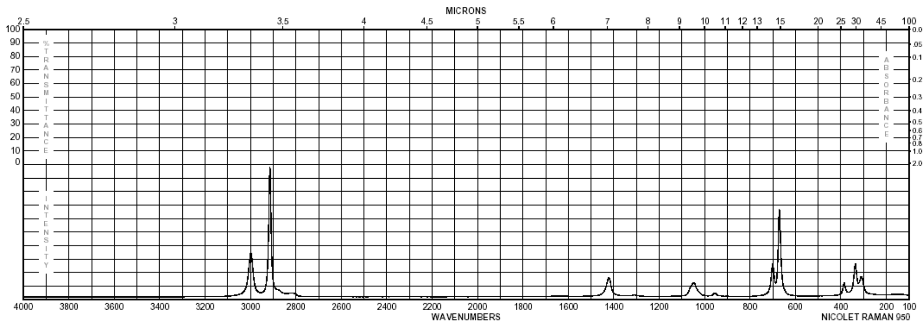
二甲亚砷
