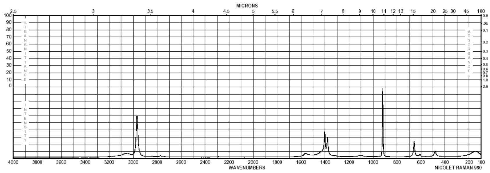
硝基甲烷
