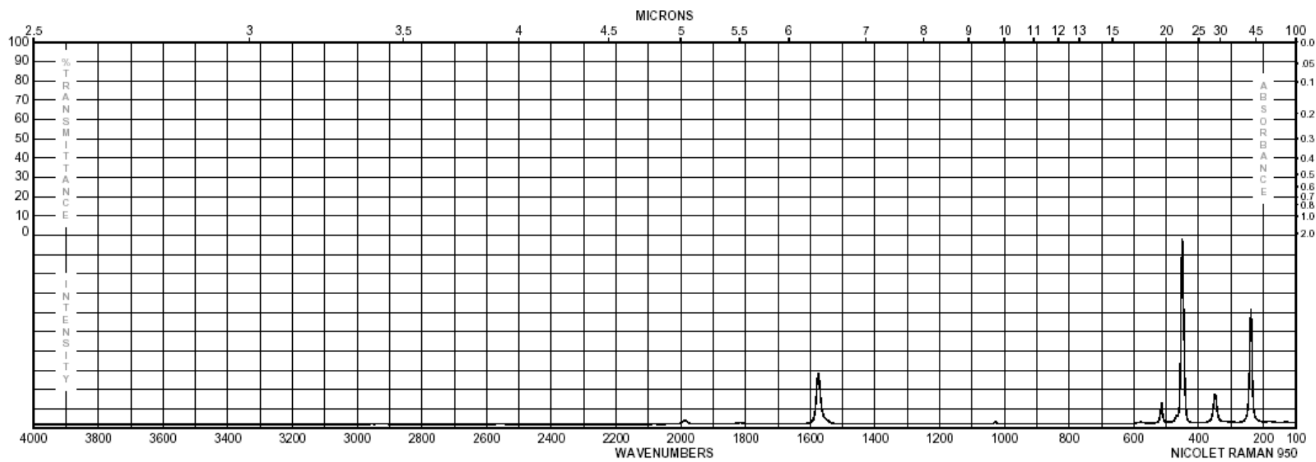
四氯乙烯
