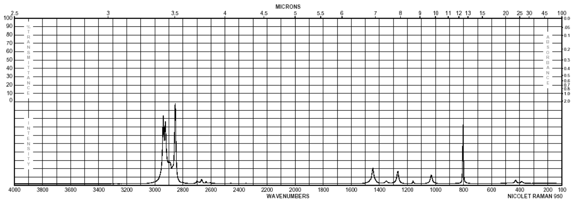
环己烷
