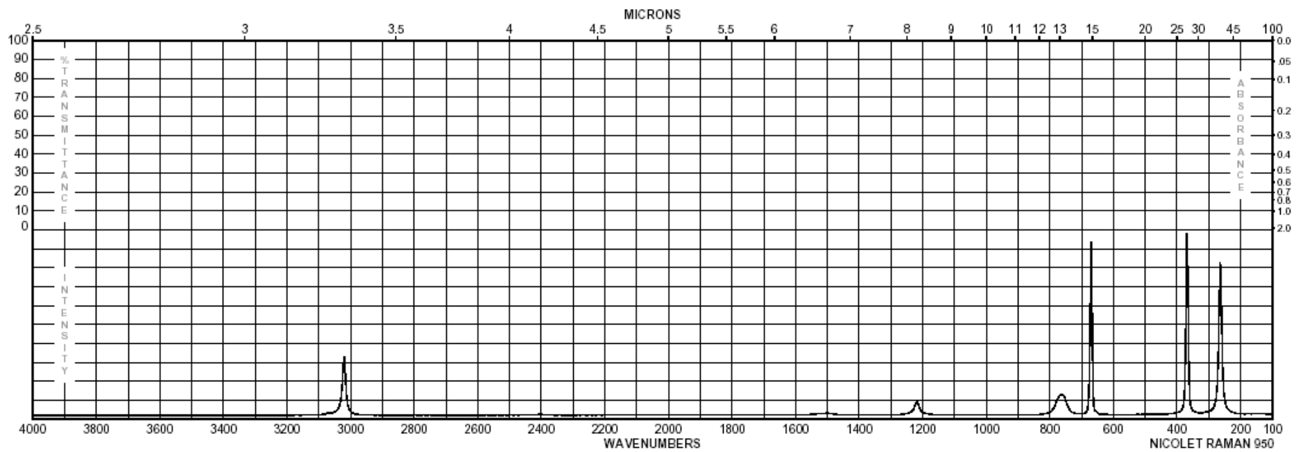
三氯甲烷
