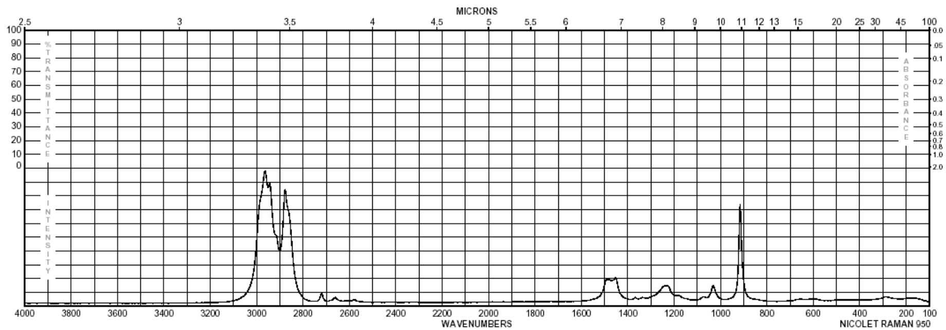
四氢吲哚
